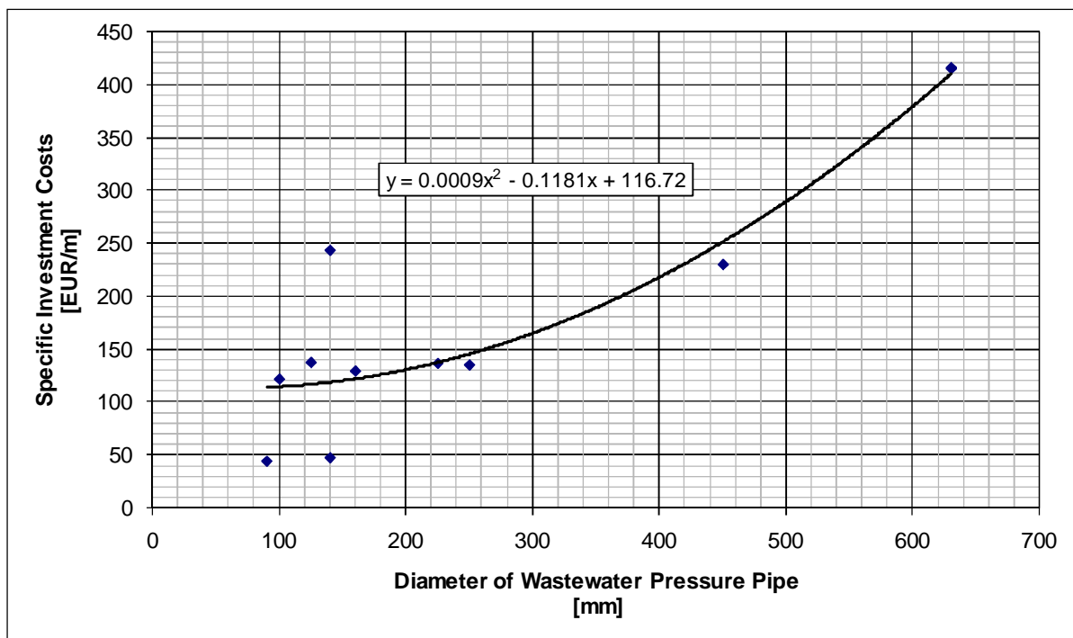
Figura 7.4-8: Diametrul conductei de presiune
