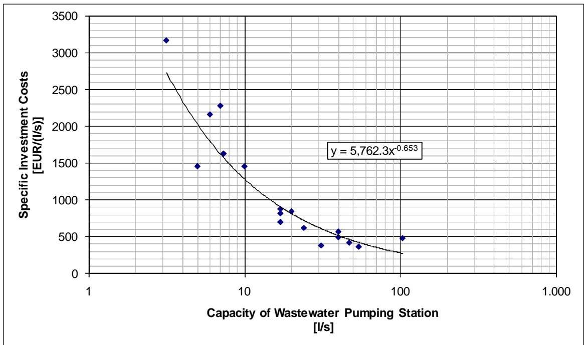
Figura 7.4-7: Capacitatea pompei
