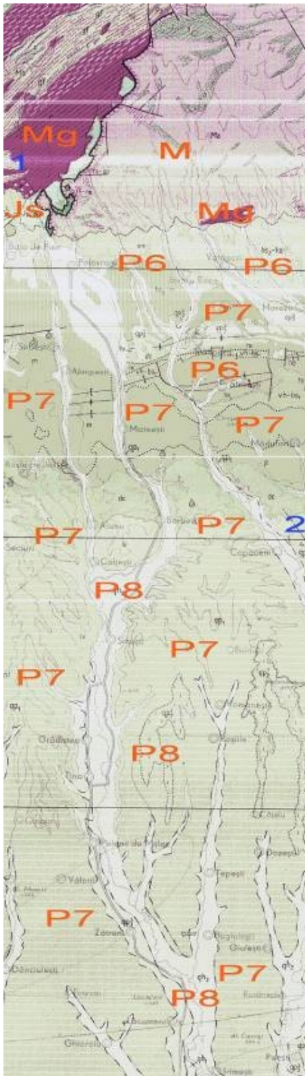
Fig. 2.3- 1: Unitati Geologice – Bazinul Oltului
