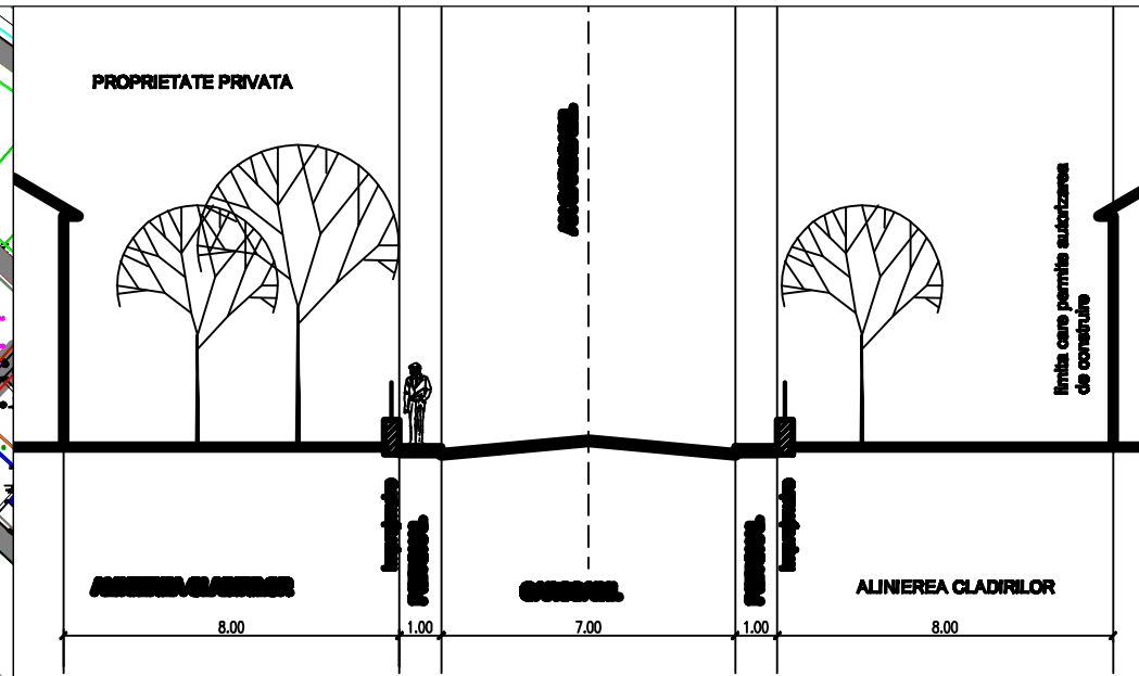
PROFIL TRANSVERSAL AA
